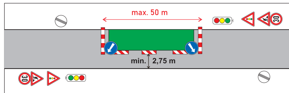
OZNAČENÍ PRACOVNÍHO MÍSTA V NEPŘEHLEDNÉM ÚSEKU
