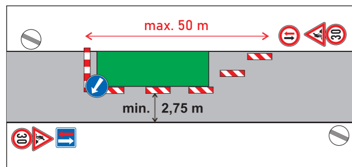
OZNAČENÍ PRACOVNÍHO MÍSTA V NEPŘEHLEDNÉM ÚSEKU
