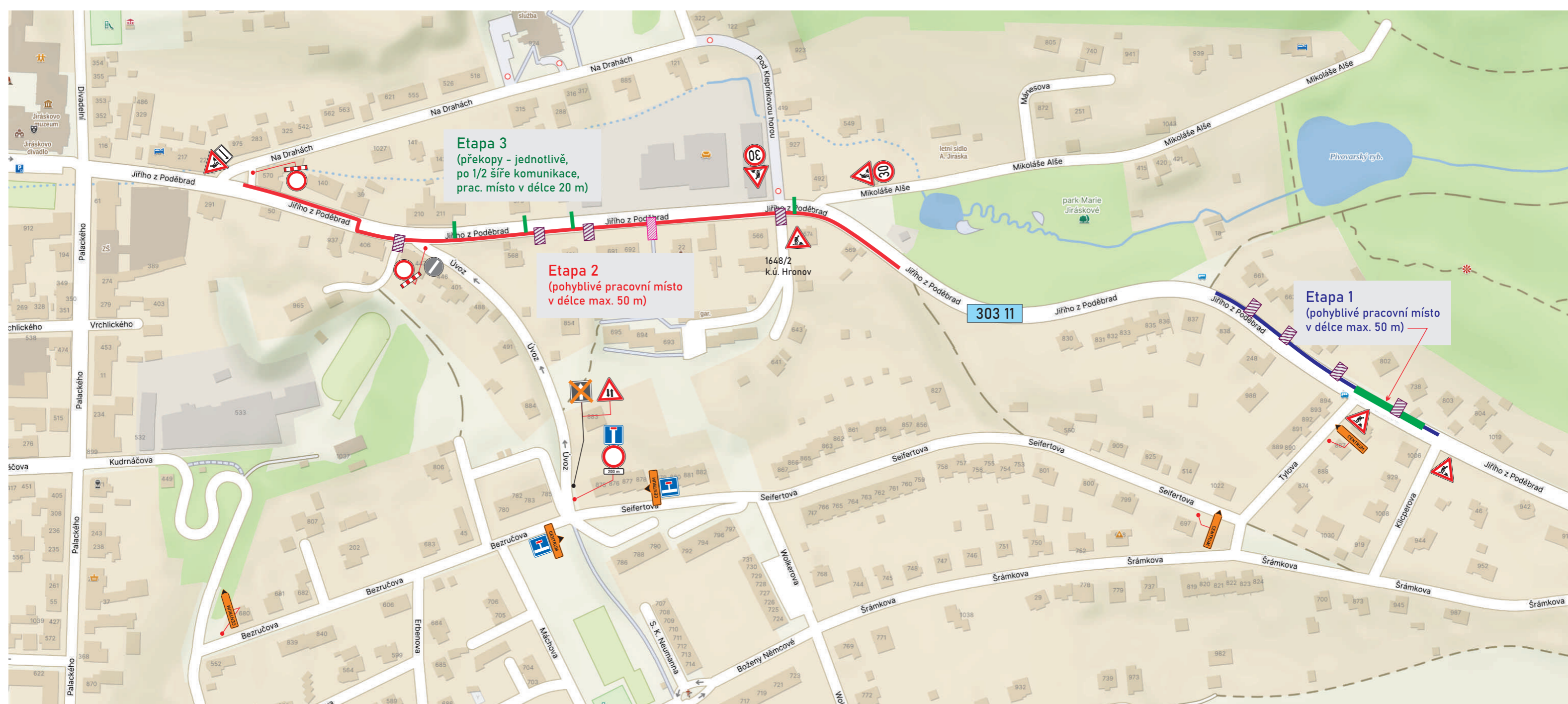
OZNAČENÍ PRACOVNÍHO MÍSTA V PŘEHLEDNÉM ÚSEKU
